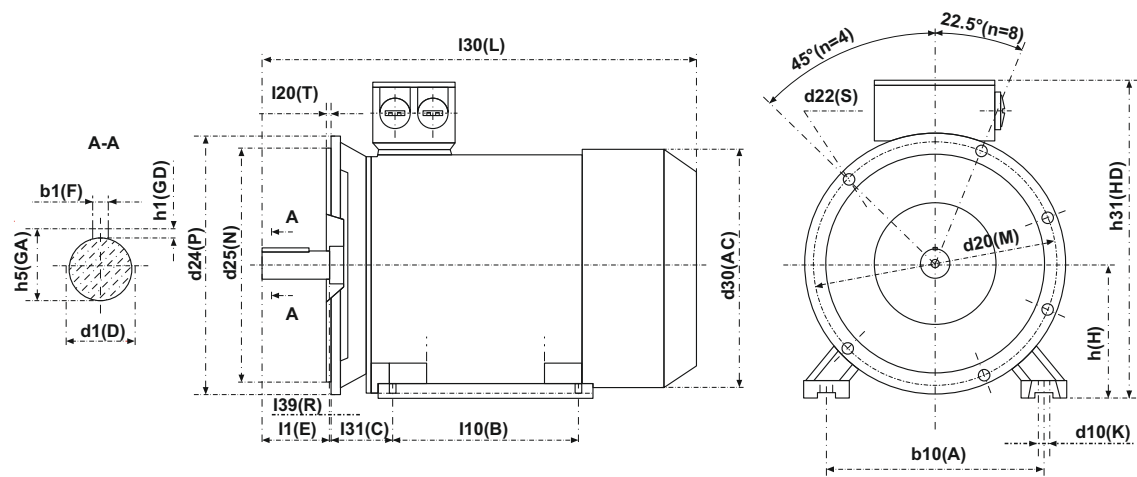
Монтажное исполнение IM 20..1
