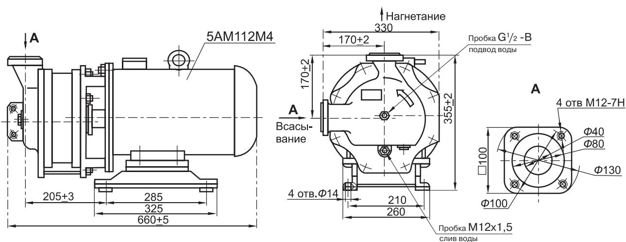
Электронасос ВВН1-1,5
