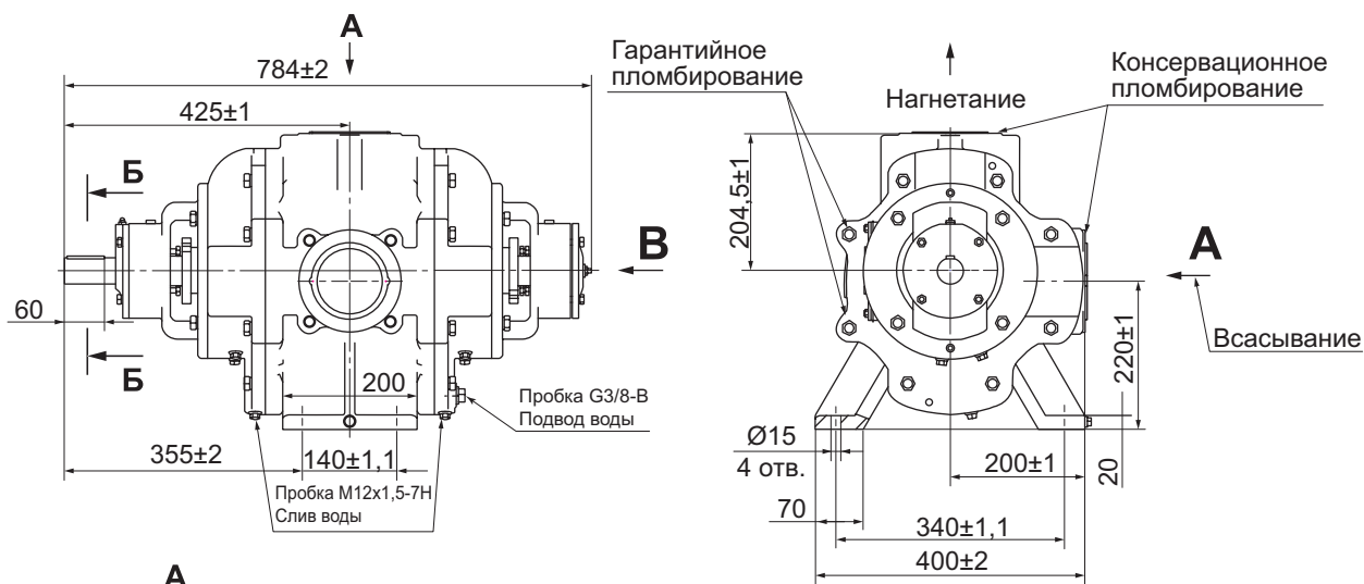
Насос ВВН1-6
