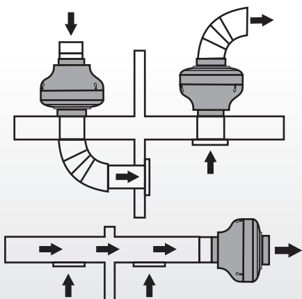
Примеры монтажа в вентиляционные системы
